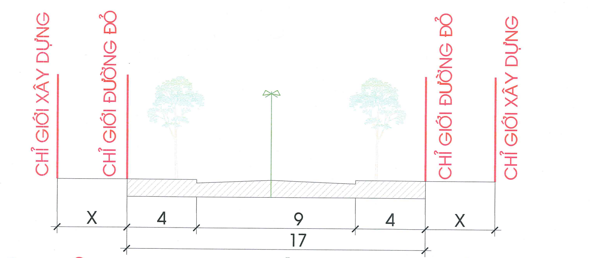
MẶT CẮT 2-2
