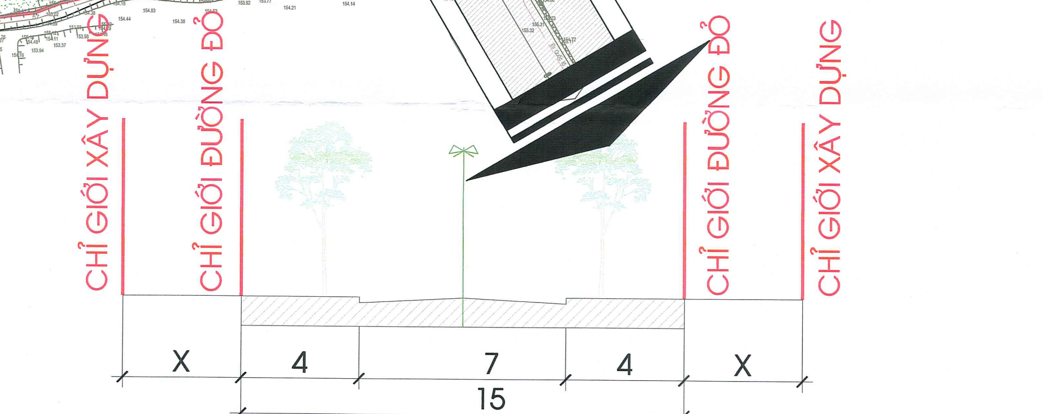
MẶT CẮT CÁC TUYẾN ĐƯỜNG NỘI KHU CỦA TOÀN DỰ ÁN
